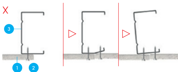
ONJUISTE volgorde van bevestiging aan stalen profiel.
