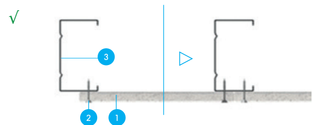
JUISTE volgorde van bevestiging aan stalen profiel.
